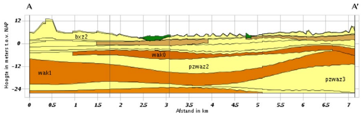
Figuur 7-1 Bodemopbouw langs tracé
