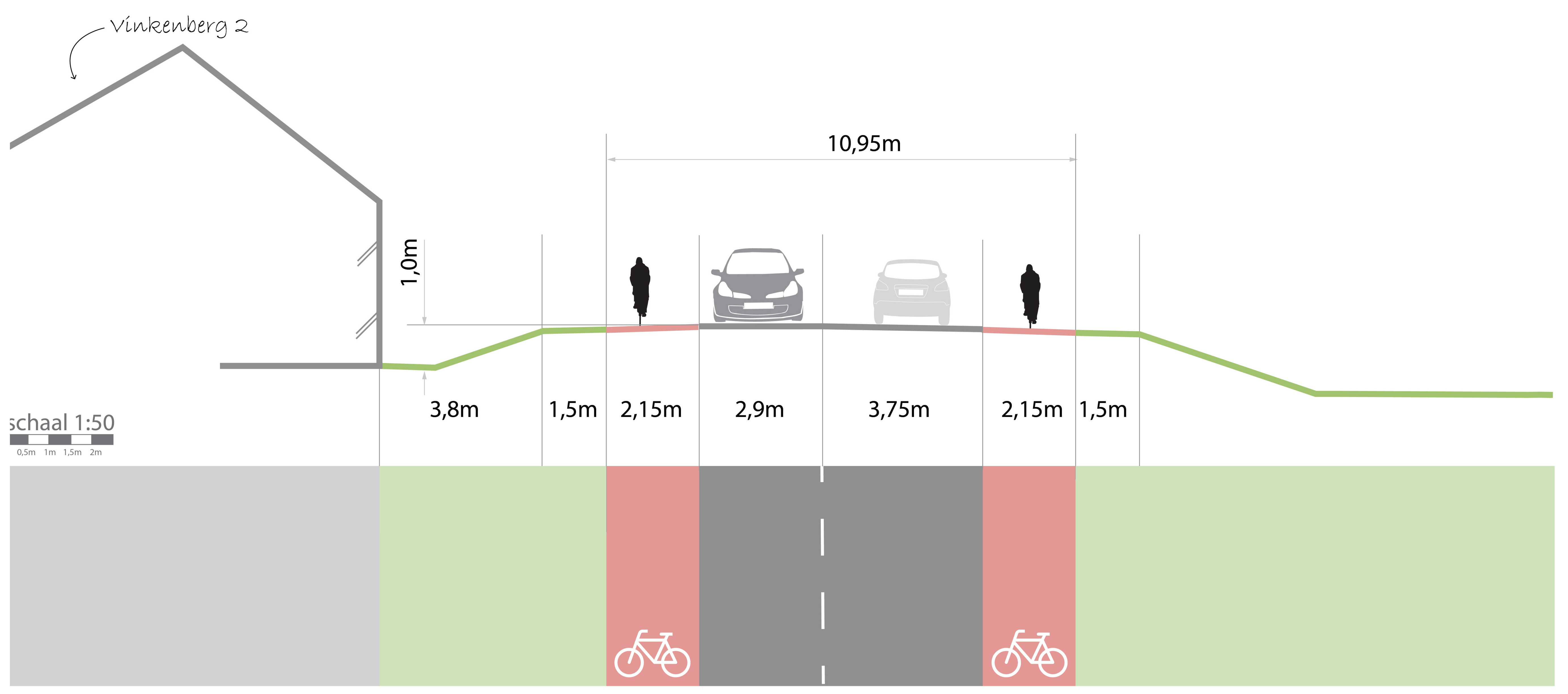
Doorsnede II
